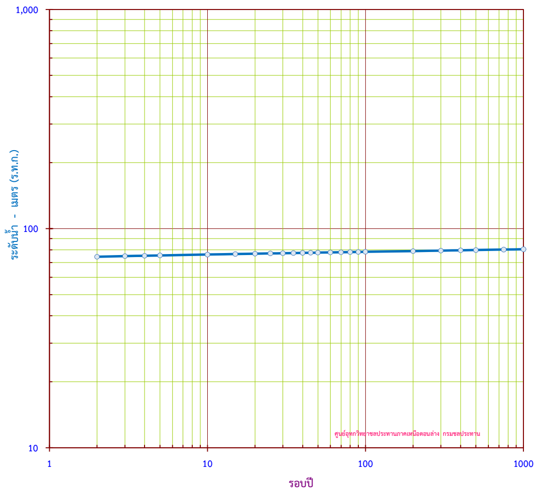
กราฟแสดง ระดับน้ำสูงสุดรายปี ขนาดรอบปีต่างๆ สถานี P.7A อ.เมือง จ.กำแพงเพชร
